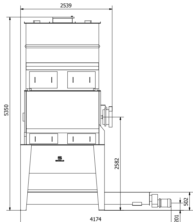
3-pași - mixer + pre-cuvă + cuvă descărcare
